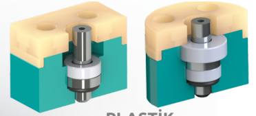
PLASTİK İŞ PARÇALARI (100 takım)
