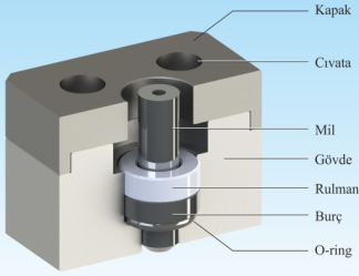
İŞ PARÇASI ELEMANLARI
